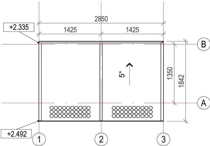
Jumta plāns 1 : 50
