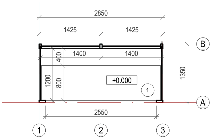
1. stāva plāns 1 : 50
