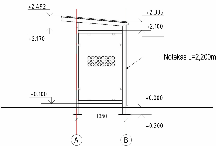
Fasāde asīs A-B 1 : 50
