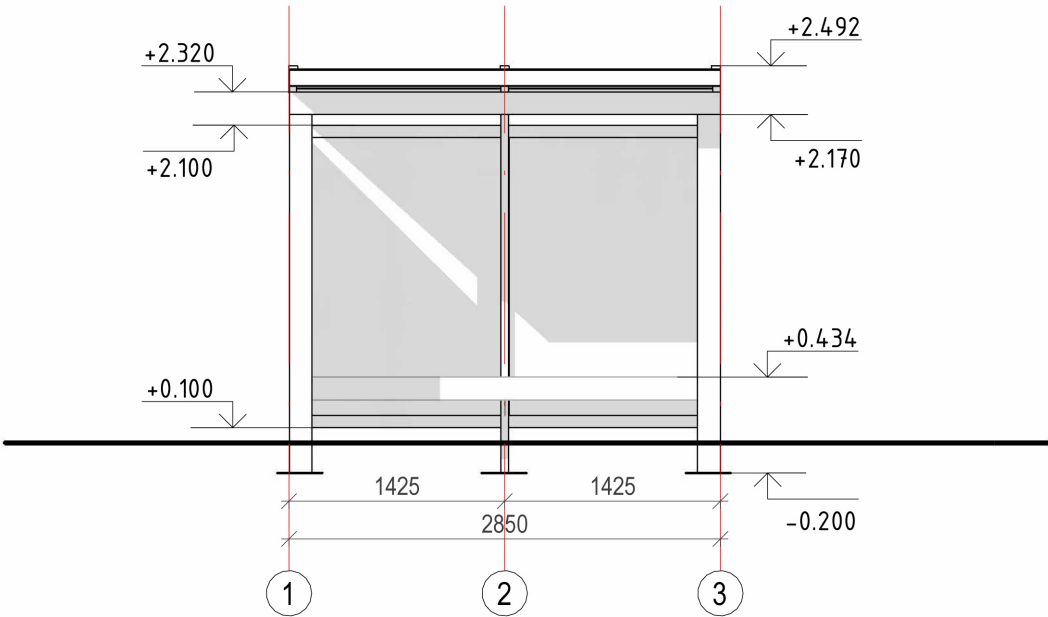
Fasāde asīs 1-3 1 : 50
