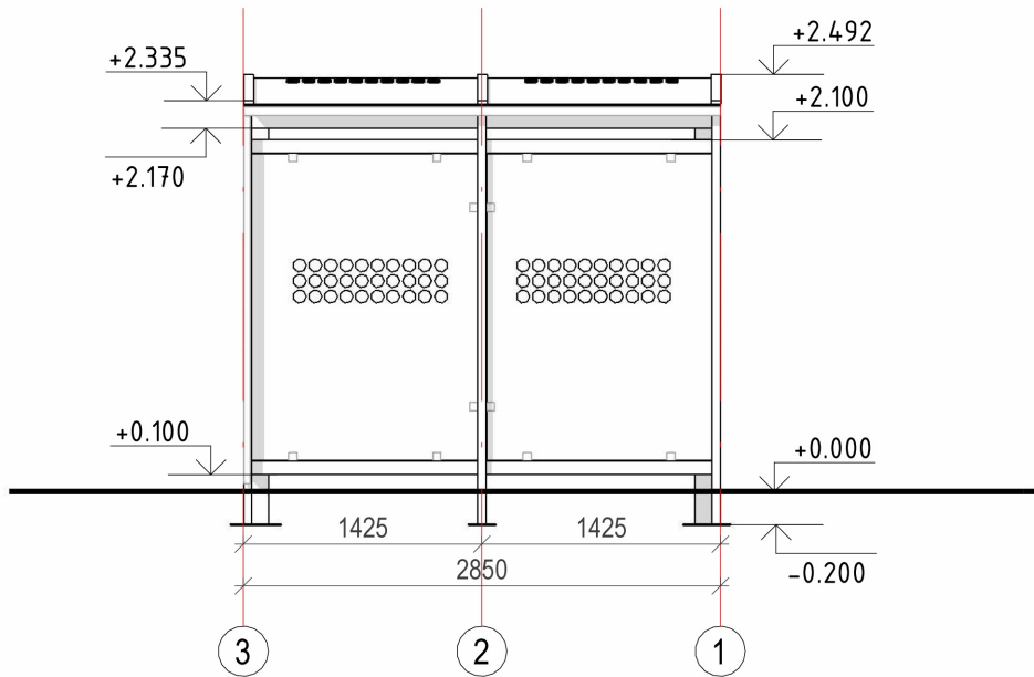
Fasāde asīs 3-1 1 : 50
