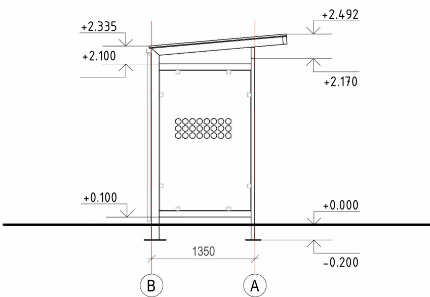
Fasāde asīs B-A 1 : 50
