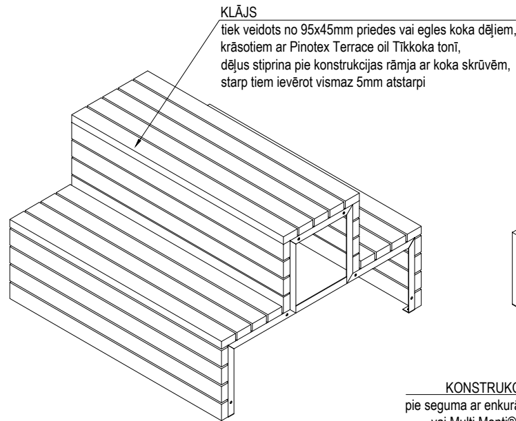
AKSONOMETRIJA
