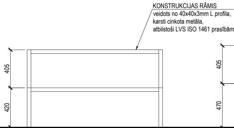
SĀNSKATS KONSTRUKCIJAS RĀMIM M 1:25
