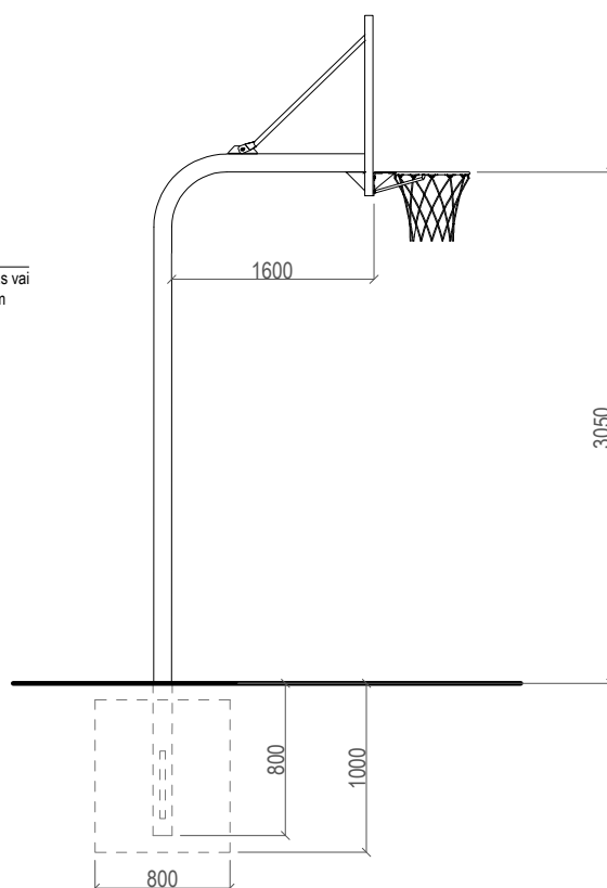
SĀNSKATS M 1:50
