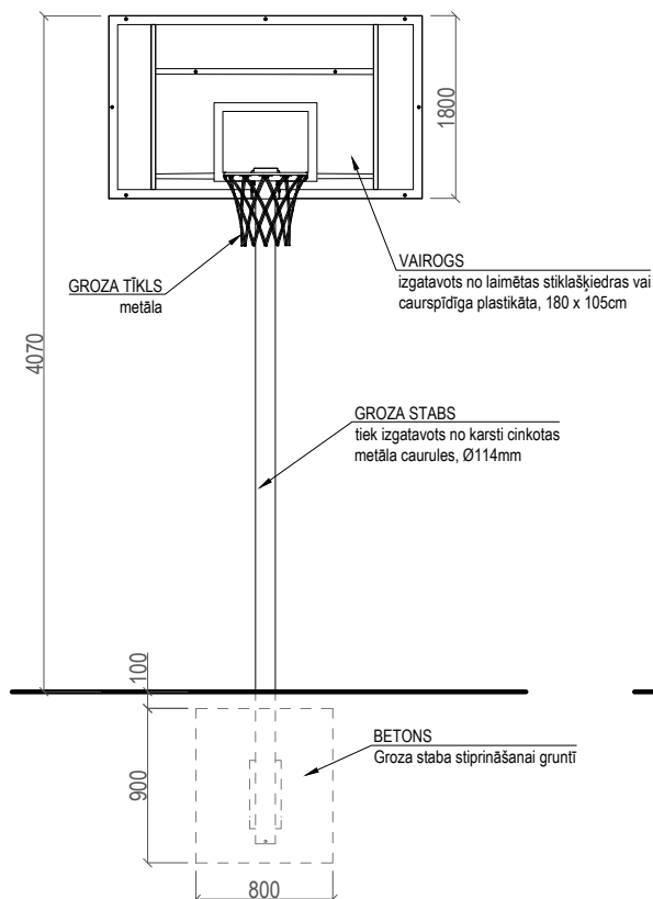
PRETSKATS M 1:50
