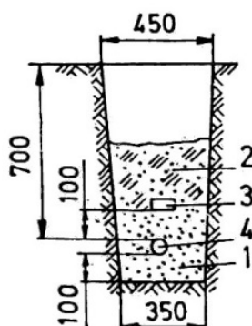
7.11-1 attēls. Kabeļu/kanalizācijas guldīšanas shēma
