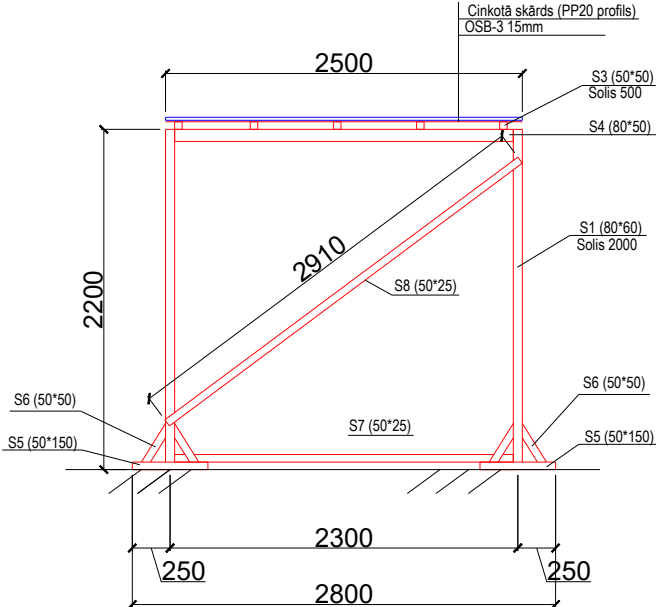
Griezums A-A
