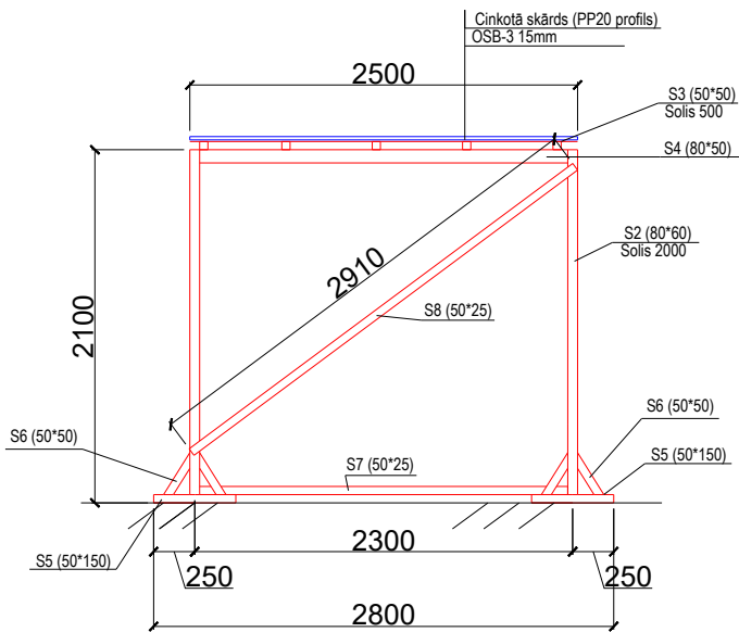
Griezuma B-B
