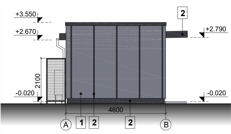
Fasāde asis A-B
