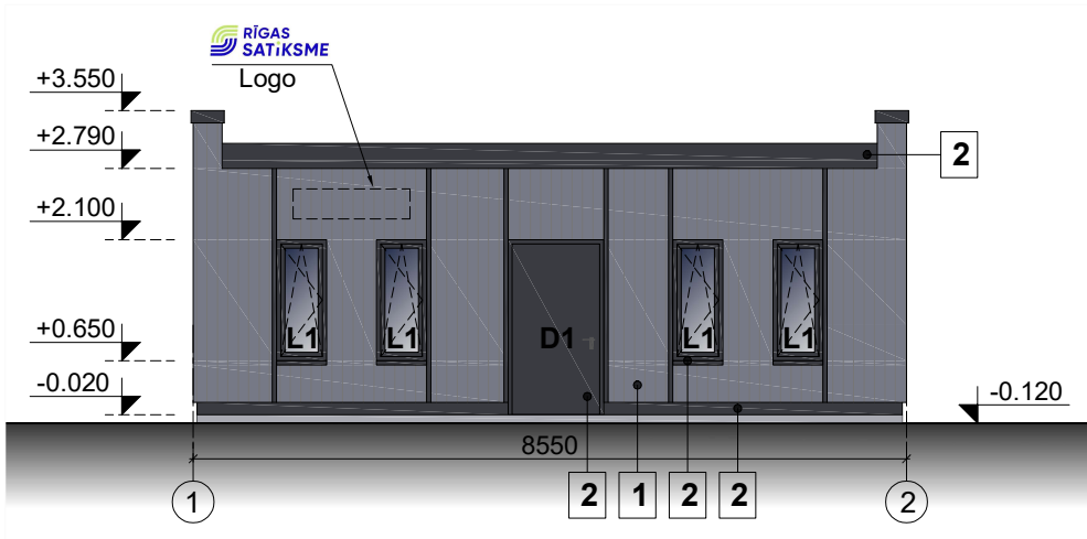
Fasāde asis 1-2 (Galvenā fasāde)
