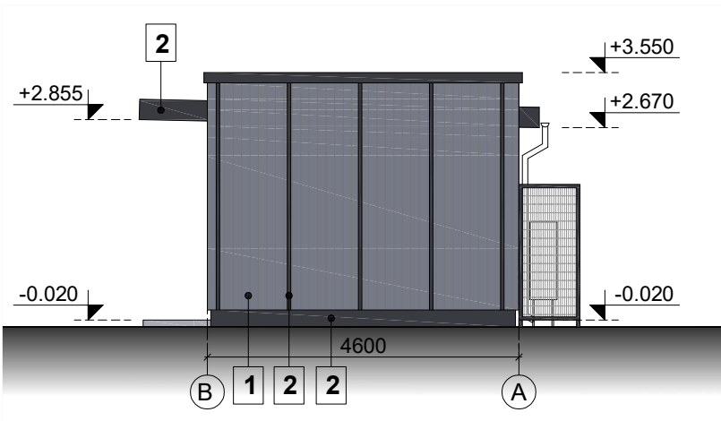
Fasāde asis B-A
