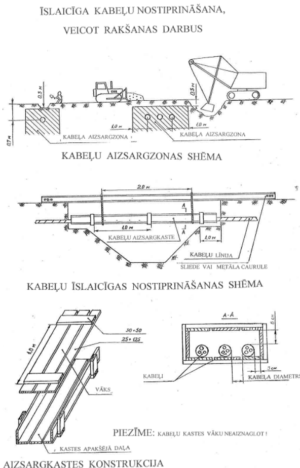
1.att. – kabeļu nostiprināšana, veicot rakšanas darbus
