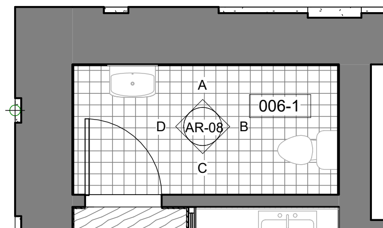
Telpas 006-1 grīdas plāns M 1 : 50
