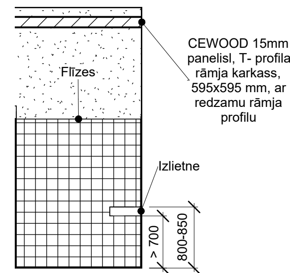
Telpas 006-1 sienas notinums D M 1 : 50
