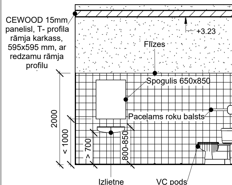
Telpas 006-1 sienas notinums A M 1 : 50
