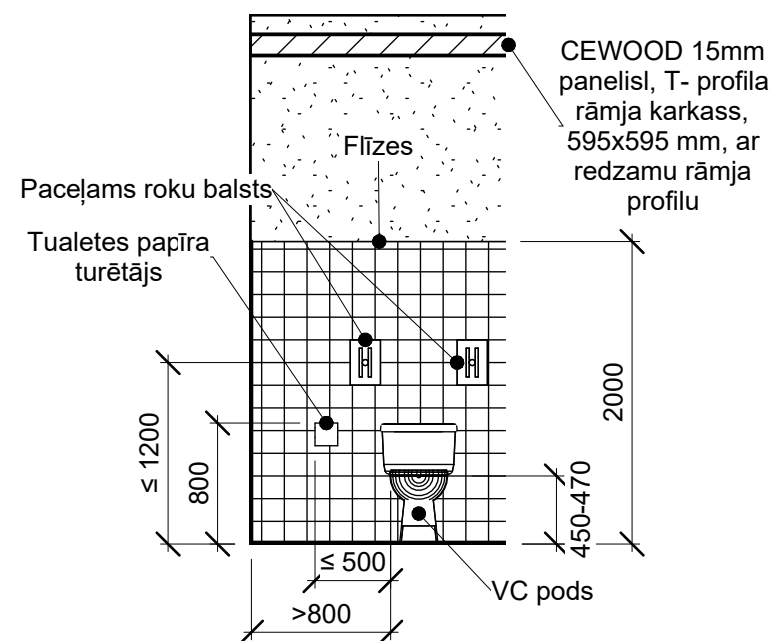
Telpas 006-1 sienas notinums B M 1 : 50
