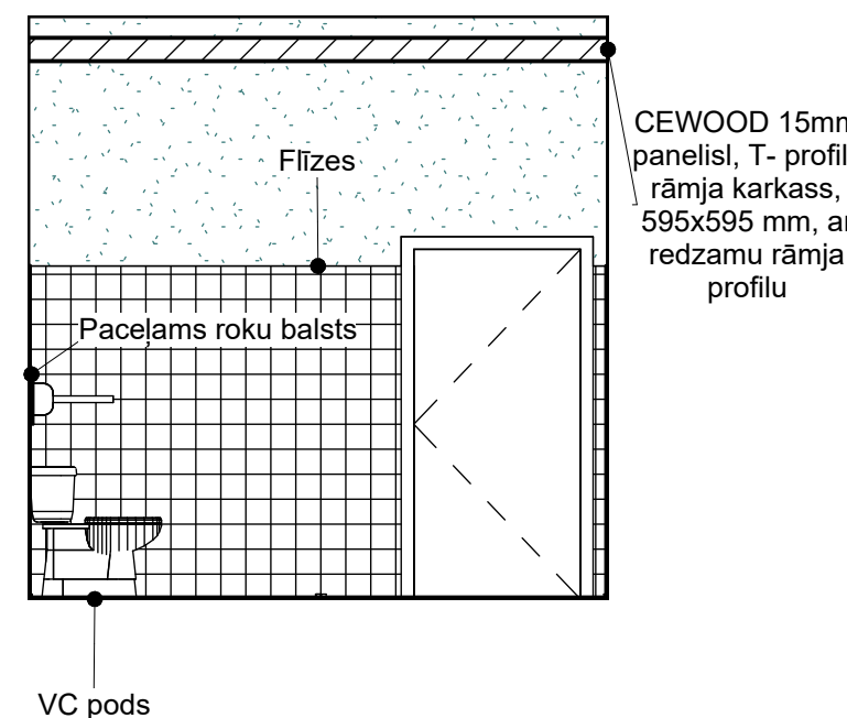
Telpas 006-1 sienas notinums C M 1 : 50
