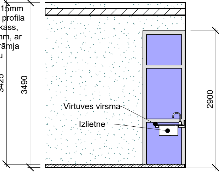
Telpas 006-2 sienas notinums D M 1 : 50
