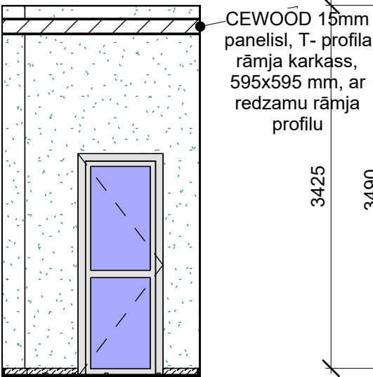
Telpas 006-2 sienas notinums C M 1 : 50
