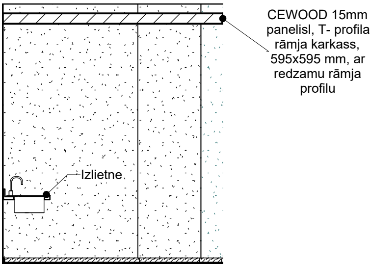
Telpas 006-2 sienas notinums B M 1 : 50
