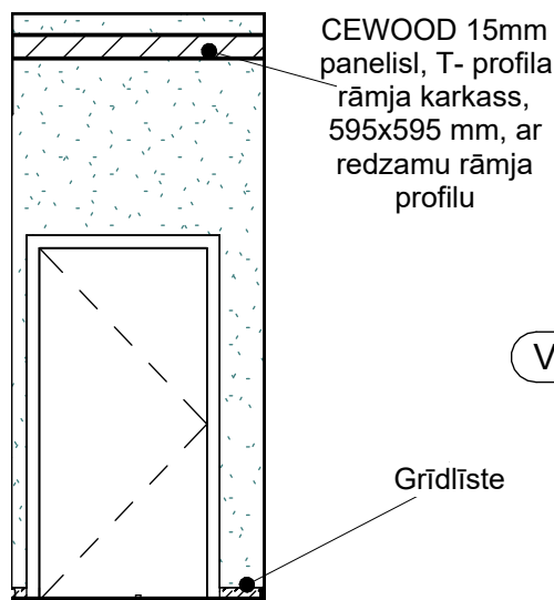
Telpas 006-4 sienas notinums A M 1 : 50
