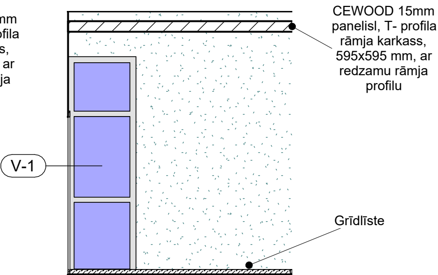
Telpas 006-4 sienas notinums B M 1 : 50
