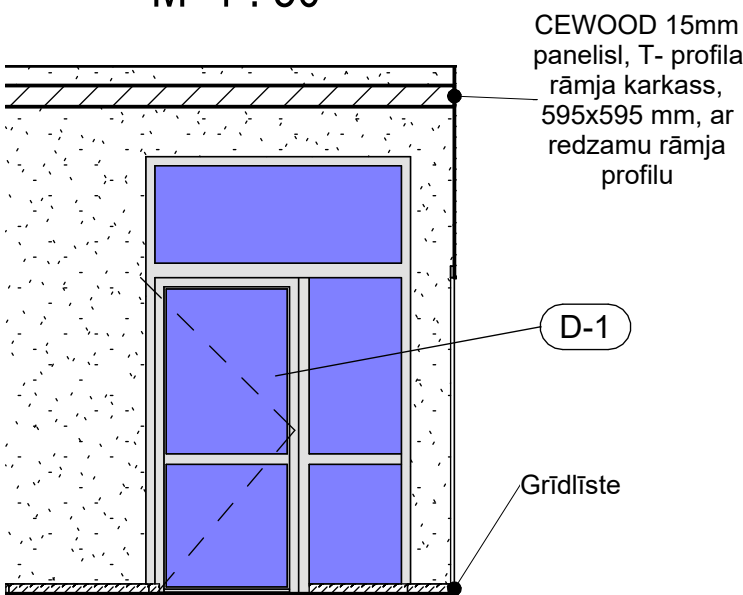
Telpas 006-4 sienas notinums D M 1 : 50
