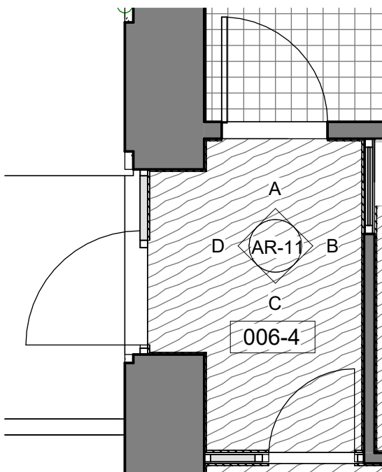
Telpas 006-4 grīdas plāns M 1 : 50
