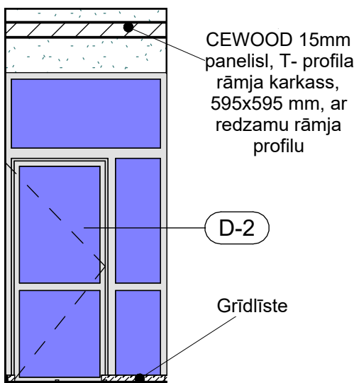
Telpas 006-4 sienas notinums C M 1 : 50
