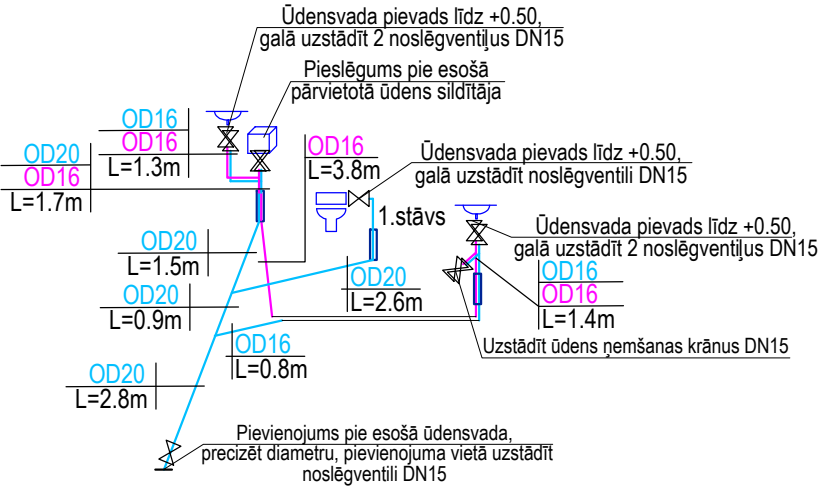
Iekšējā ūdensvada aksonometrija
