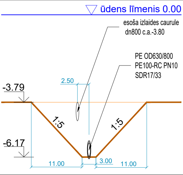
15-15
