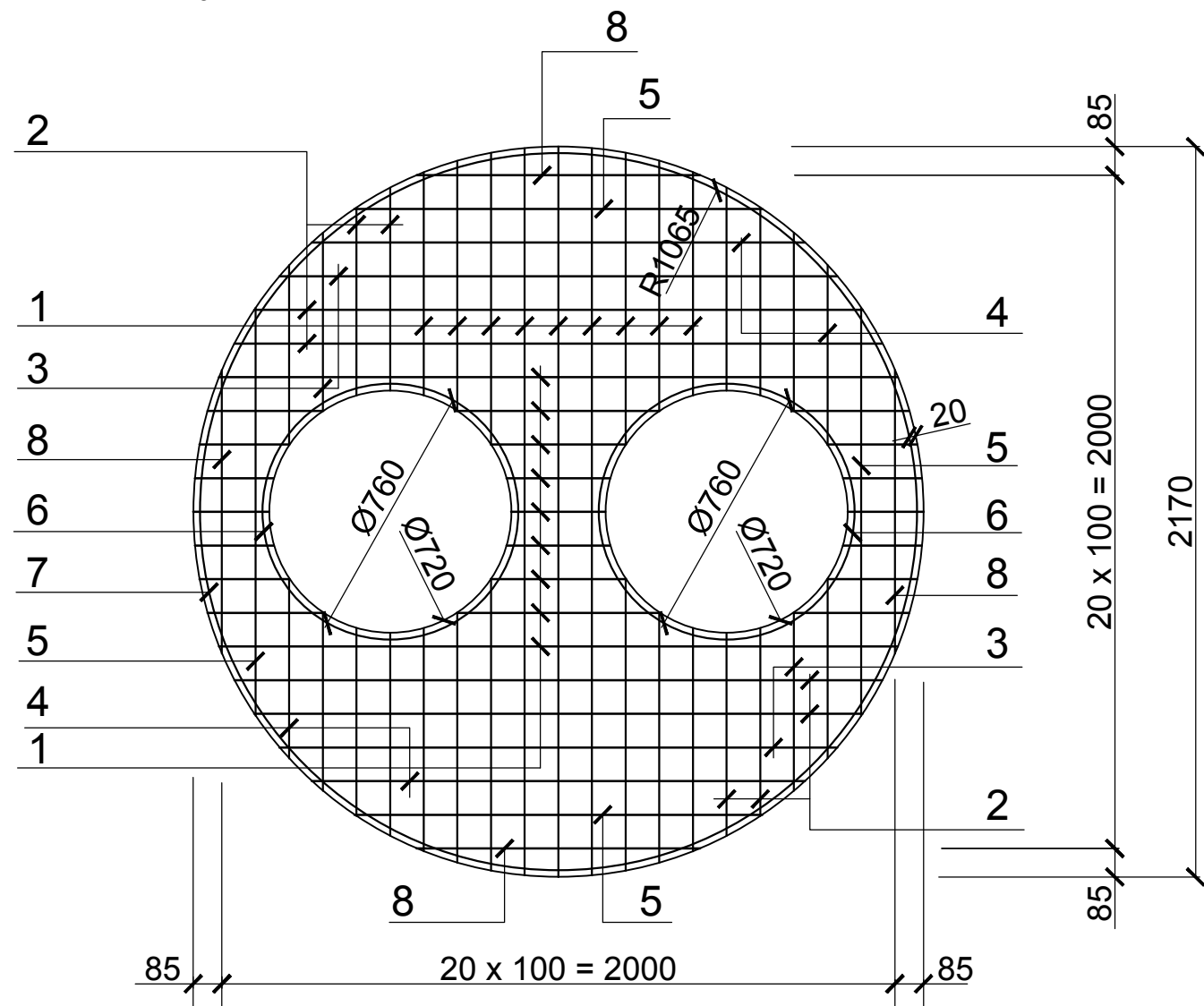
KCP-20 apakšējais un augšējais stiegru siets St-1 M 1:20
