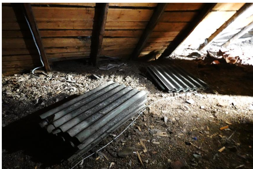
Skats uz vienu no ēkas A korpusa slīpnēm ar vēsturiskajām spārēm un no jauna ieklātu dēļu klāju. Priekšplānā ap 1975. gadu jumtam uzklātās un pēdējās jumta seguma nomaiņas laikā atkal noņemtās gofrētā šifera (azbestcements) loksnes. 2025. g. foto
