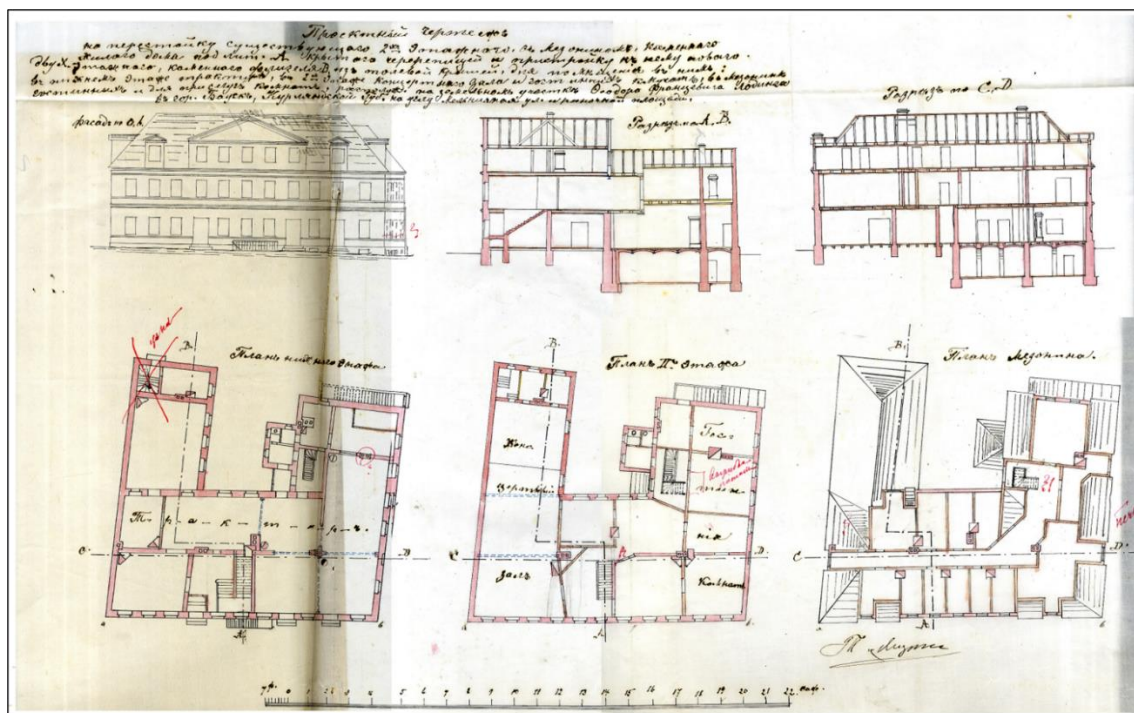
Teodora Lodinga īpašuma – viesnīcas – pārbūves projekts, pirms 1900. g. LNA LVVA, 97. fonds, 1. apraksts, 770. lieta, 2. lpp.
