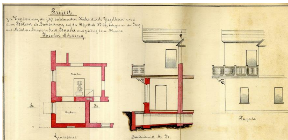
Virtuves paplašināšanas projekta lapa. 1904. gads.
