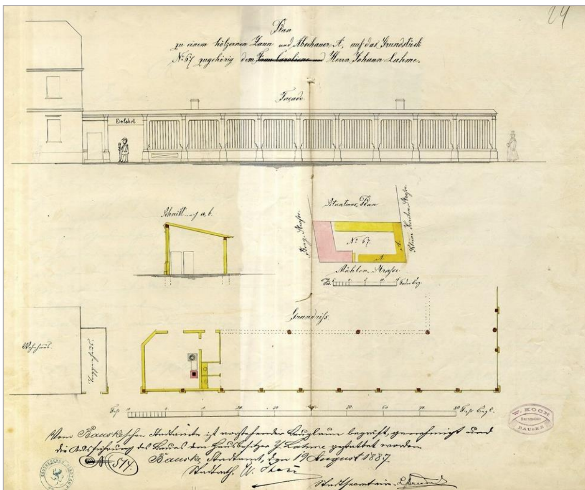
Koka žoga ar nojumi projekts Kalna ielas 6 pagalmā. 1887. LNA LVVA, 751. fonds, 2. apraksts, 287. lieta, 24. lp.
