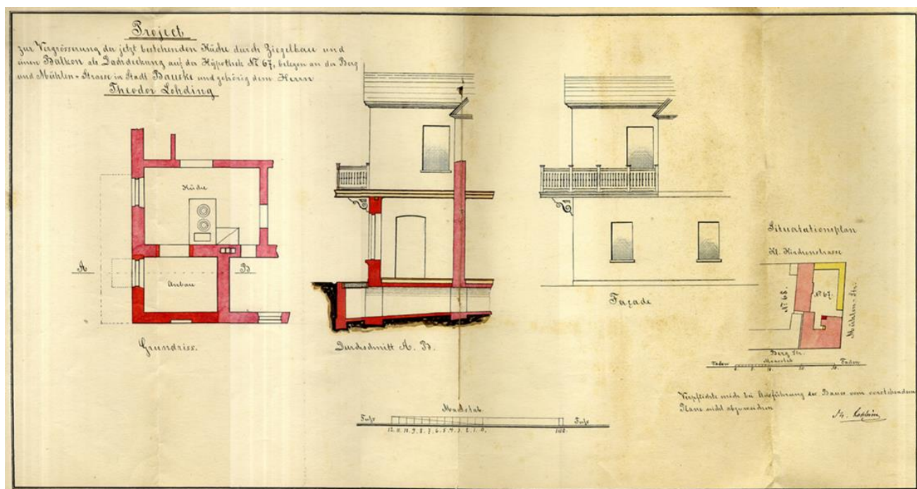
Projekts viesnīcas virtuves paplašināšanai un balkona izbūvei. 1902. g.
