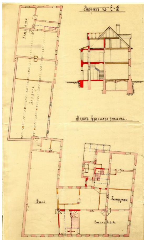
Ēkas uz gruntsgabala Nr.67, Bauska. Staļļa un ratnīcas projekts. 1900. LNA LVVA, 97. fonds, 1. apraksts, 770. lieta
