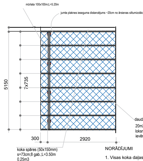
NOJUMES SPĀRU PLĀNS
