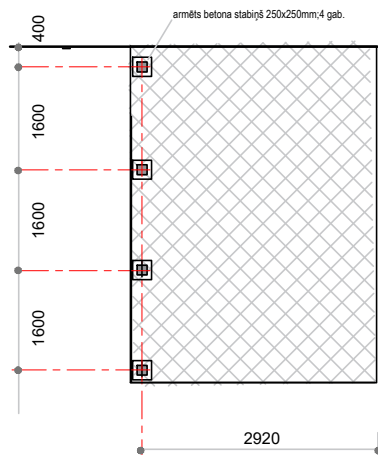
NOJUMES STATŅU PAMATU PLĀNS
